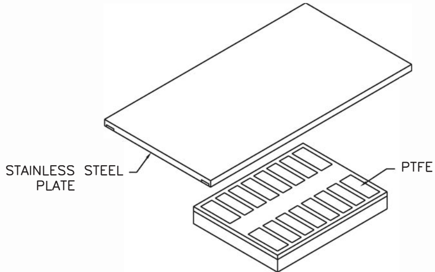
पी. टी. एफ़. ई. बेयरिंग PTFE BEARING
