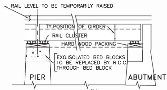
कट उद्दिष्ट SECTIONAL ELEVATION
