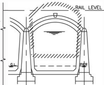
आंशिक काट उद्दिष्ट PART SECTIONAL ELEVATION
