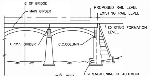
अर्ध काट HALF SECTION
