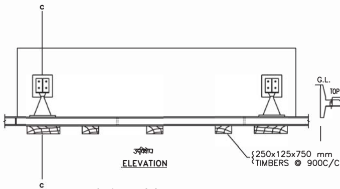
पूर्ण दलित आर.सी.सी. बॉक्सों के लिए अंतरण व्यवस्था LAUNCHING ARRANGEMENT FOR PRECAST R.C.C. BOXES
