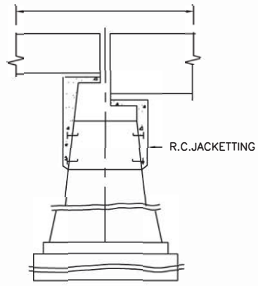
आंशिक कट उद्दिष्ट PART SECTIONAL ELEVATION
