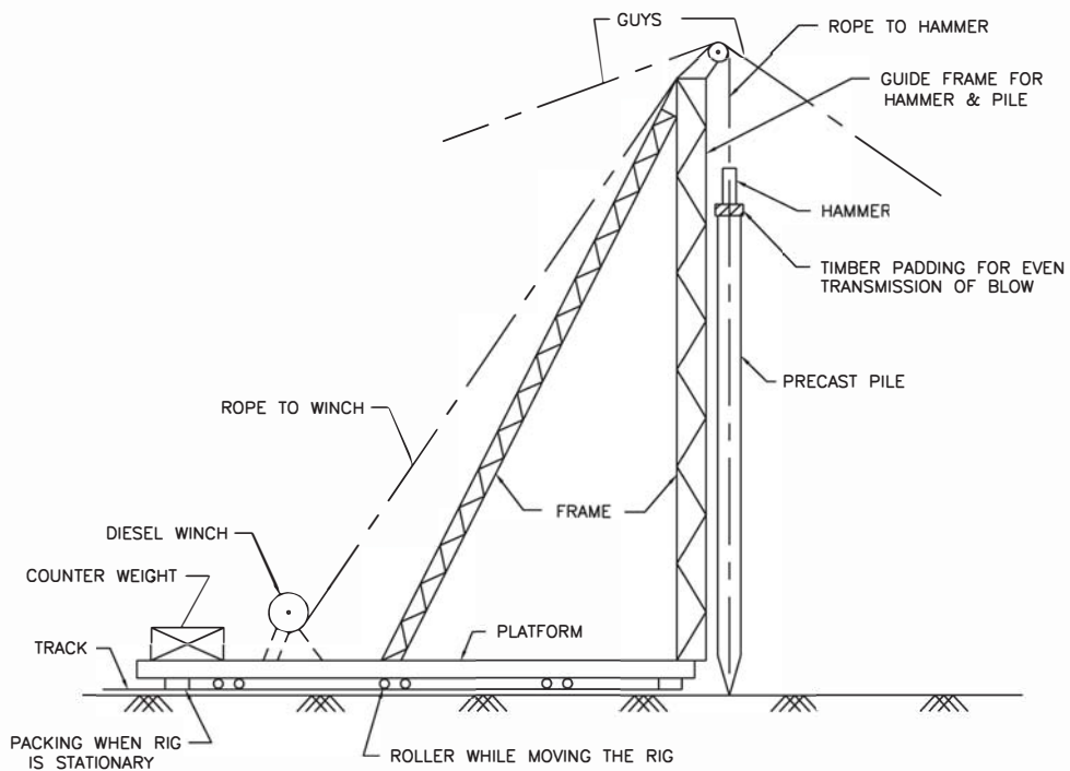
प्री ड्रॉन पाइलों को ठोकने के लिए प्रयुक्त रिग RIG USED FOR DRIVING PRE-CAST PILES
