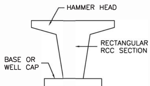
हैमर शीर्ष प्रकार का पाया HAMMER HEAD TYPE OF PIER
