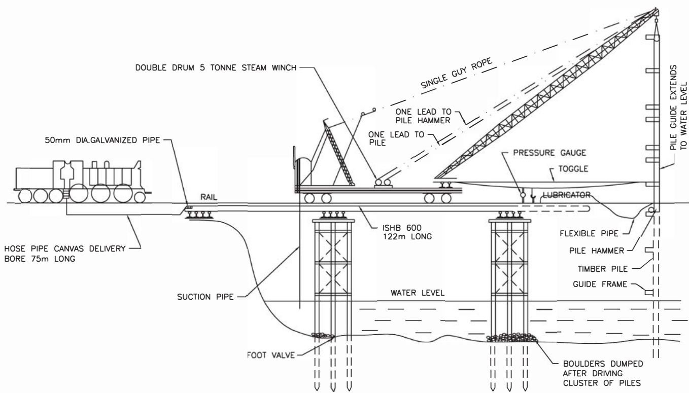
लकड़ी के पाइल वाला अस्थाई पुल TEMPORARY WOODEN PILE BRIDGE
