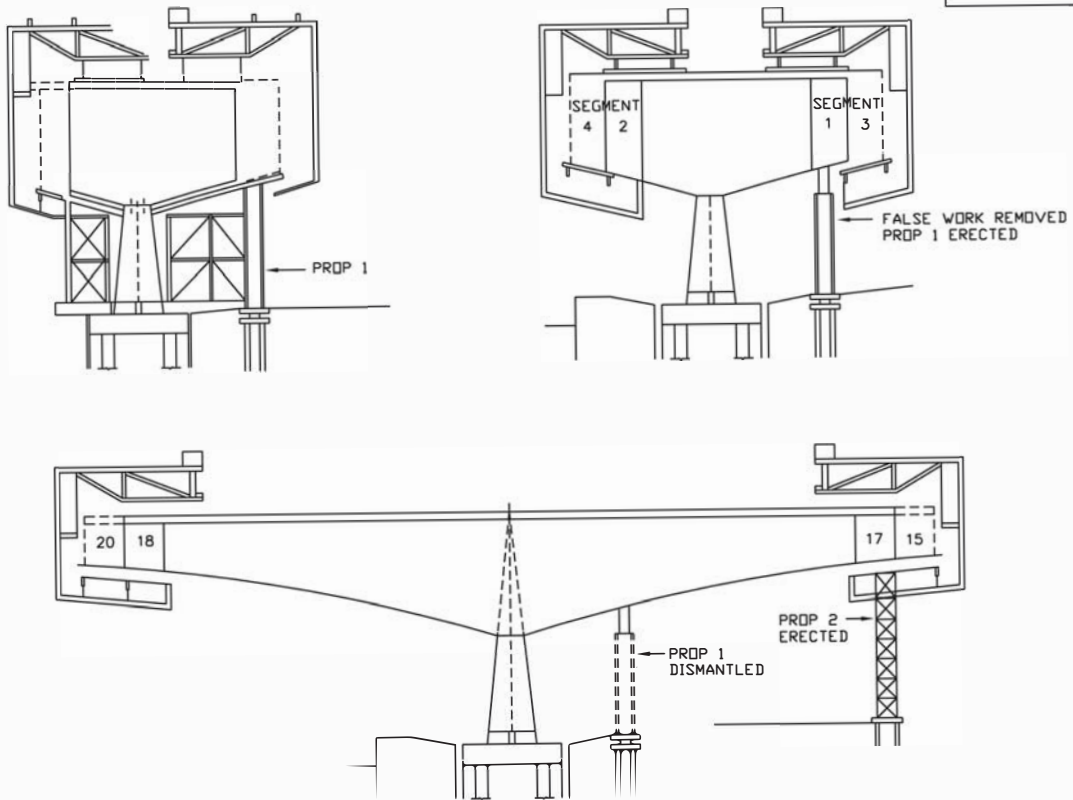
(ख) निर्माण स्थल में कैन्टीलिवर प्रणाली (b) CANTILEVER METHOD — IN SITE CONSTRUCTION
