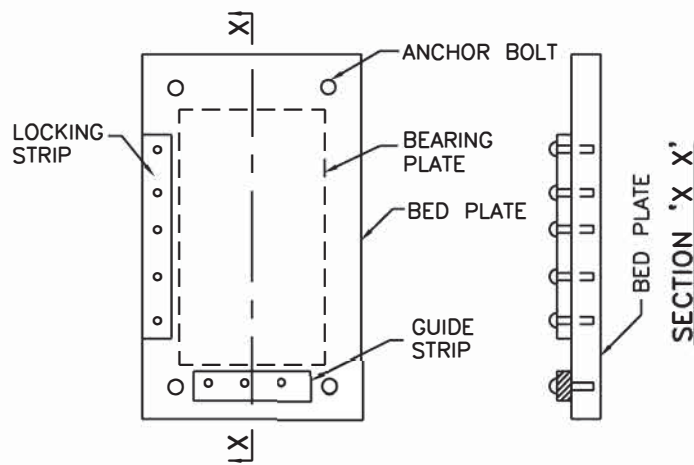
तलविशेष PLAN
