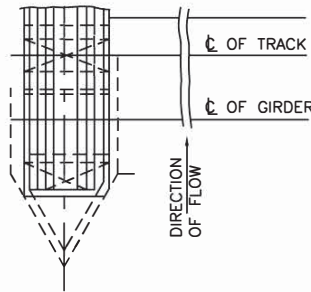
आंशिक तलविष्ट PART PLAN
