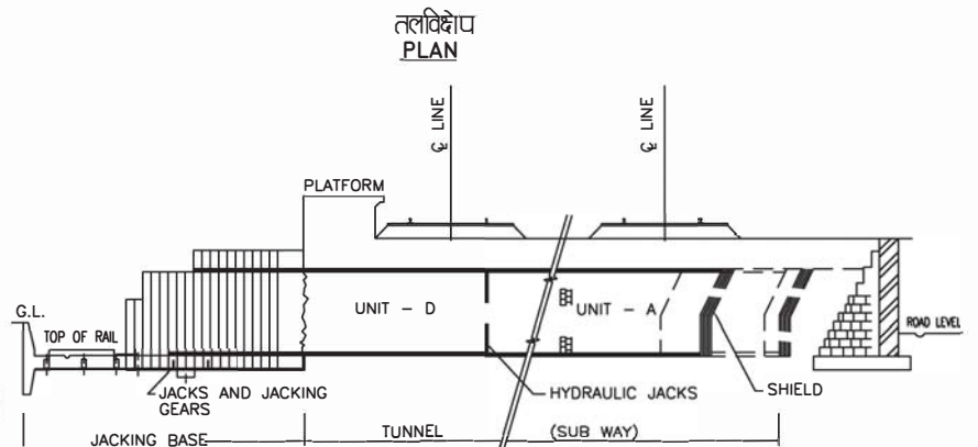
अनुबंध 5/7 पैरा 517 CROSS SECTION बॉक्स पुशिंग तकनीक BOX PUSHING TECHNIQUE
